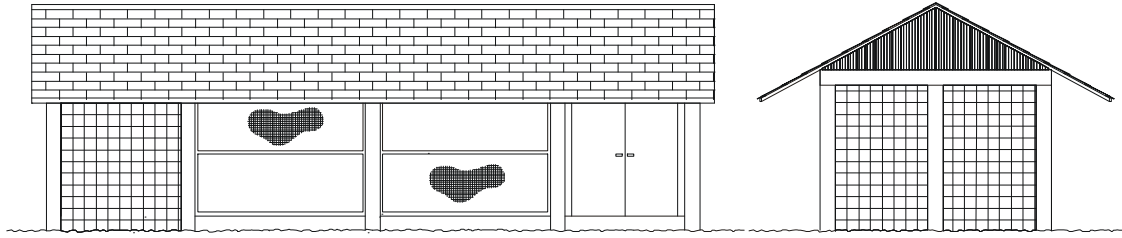
ELEVACION LATERAL
